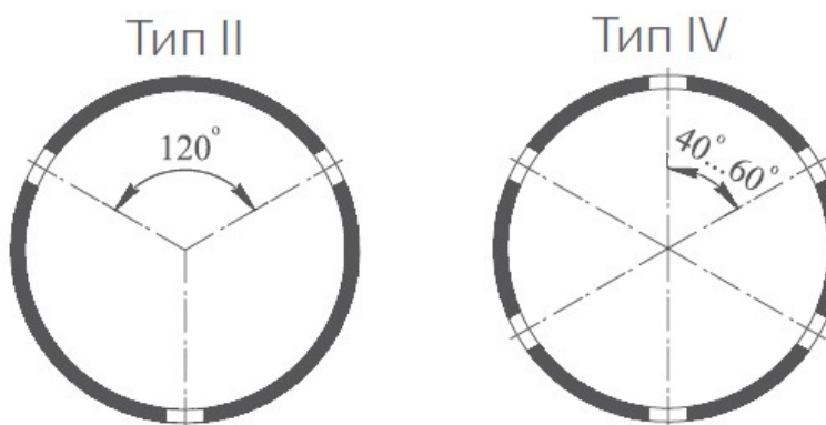
Рисунок 6 – Расположение водоприемных отверстий, полное перфорирование
