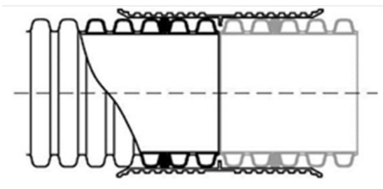
Рисунок 28 – Схема собранного муфтового соединения.
