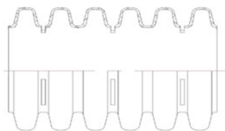
Рисунок 1 – Конструкция стенки трубы «ПЕРФОКОР ЛАЙТ»
