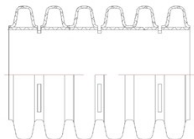
Рисунок 2 – Конструкция стенки трубы «ПЕРФОКОР» и «ПЕРФОКОР ЭКО»
