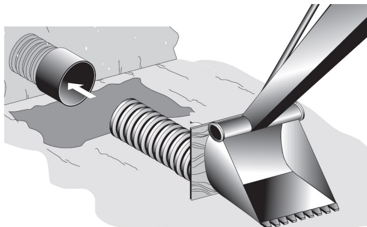
Рисунок 24 – Применение строительной техники для сопряжения труб в муфте и защита зоны соединения от загрязнения грунтом
