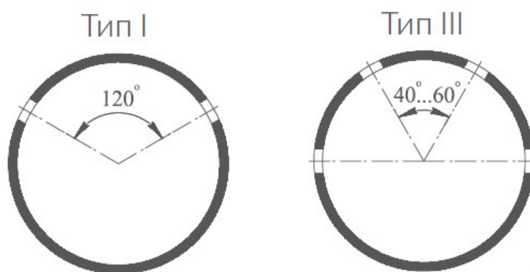
Рисунок 5 – Расположение водоприемных отверстий, частичное перфорирование
