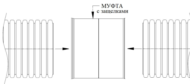
Рисунок 31 – Соединение труб ПЕРФОКОР при помощи муфт на защелках
