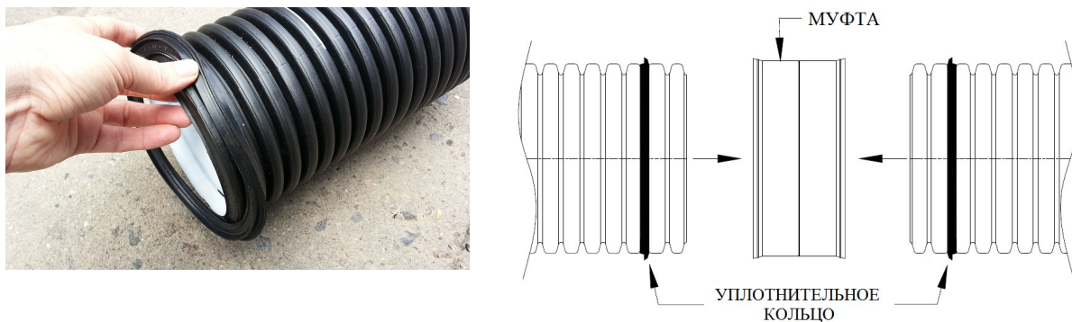
Рисунок 21 – Установка уплотнительного кольца на трубы диаметром 200 мм и менее
