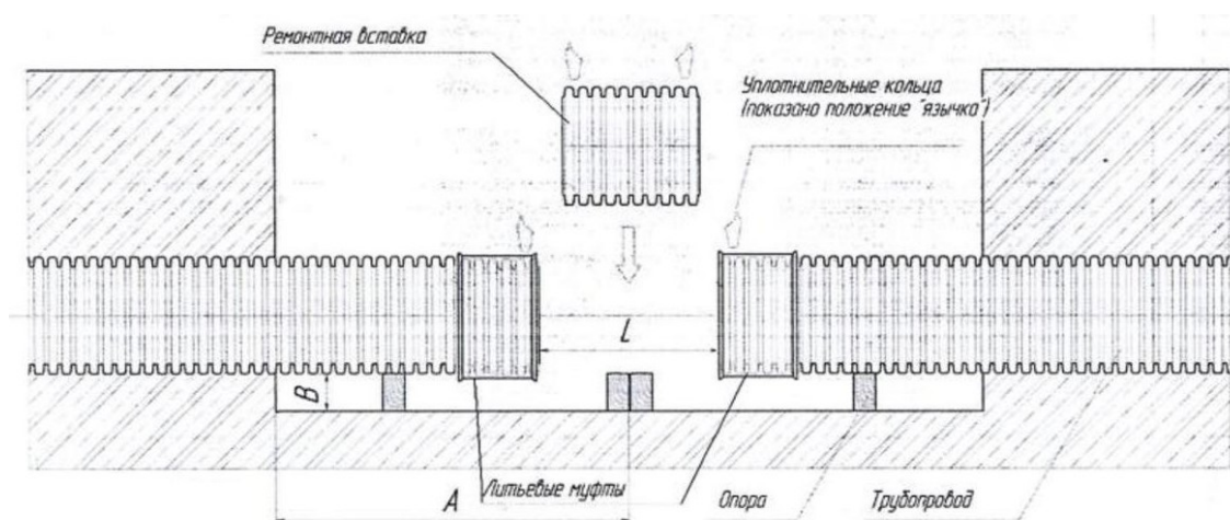
Рисунок 33 — Установка ремонтной вставки на опоры
