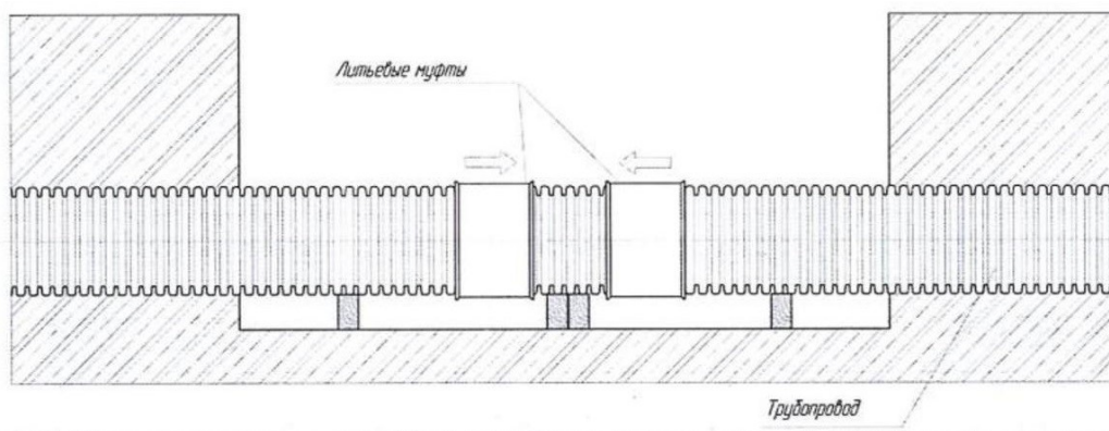
Рисунок 34 — Сборка соединений
