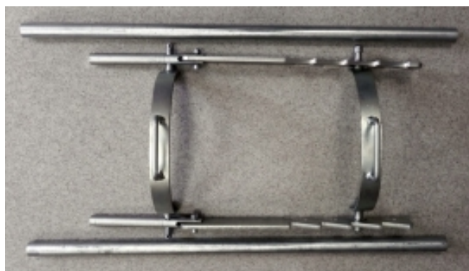
Рисунок 25 –Инструмент, применяемый для сопряжения труб ПЕРФОКОР в муфте
