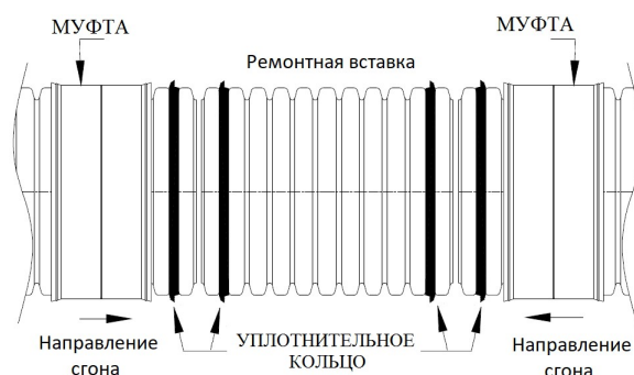
Рисунок 32 – Установка ремонтной вставки, муфт и уплотнительных колец на трубах диаметром 200 мм и менее
